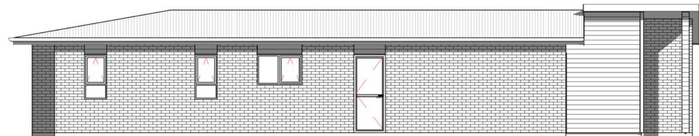
W West 1 : 100
